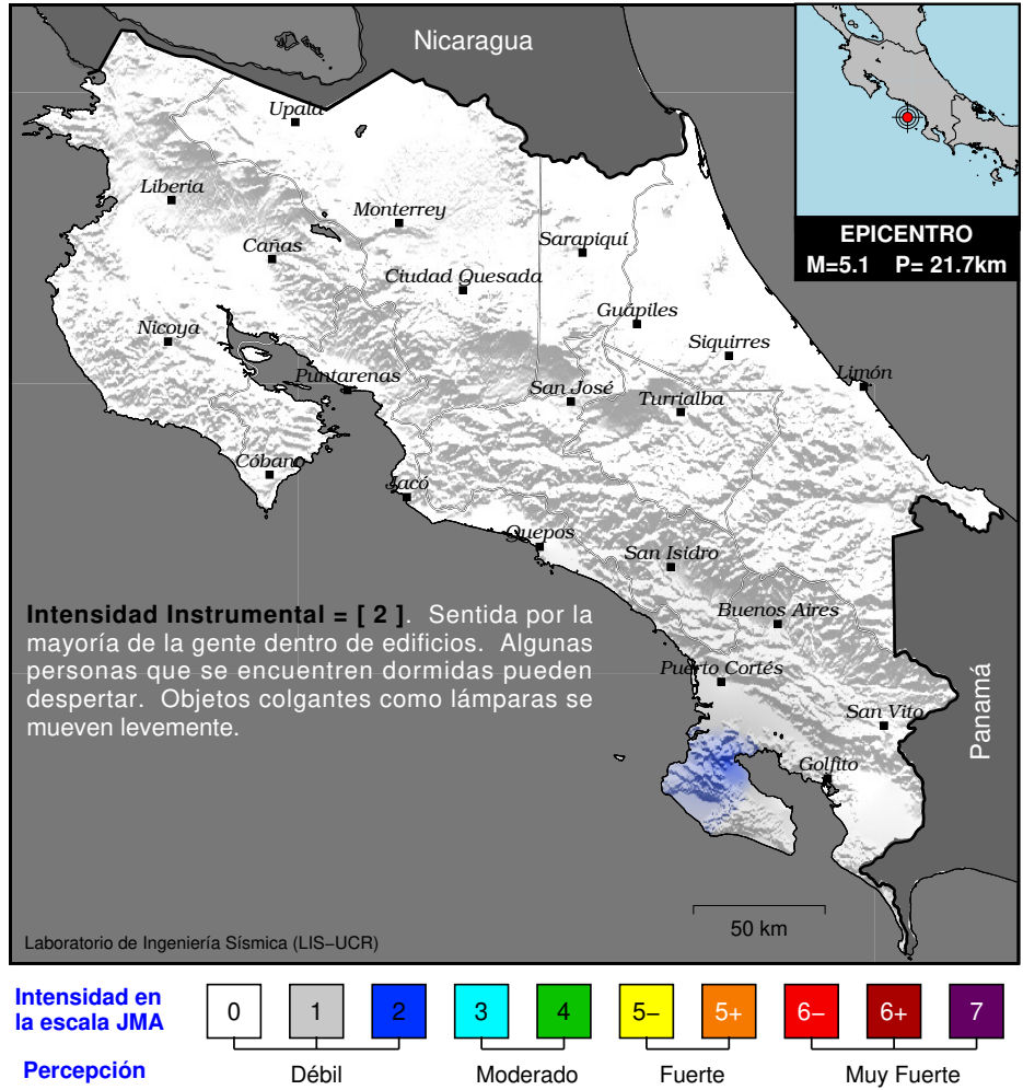
Figura 4. Mapa de intensidad JMA derivado de los valores de aceleración y duración del movimiento.
